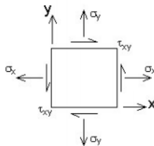
Figura 15 – Tensões no estado plano
