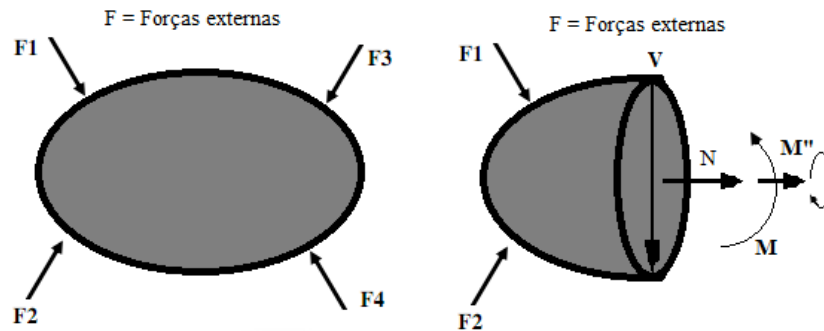
Figura 13 – Método das seções. F = forças externas; N = força normal; M = esforço torção; M'' = esforço fletor; V = força cortante.
