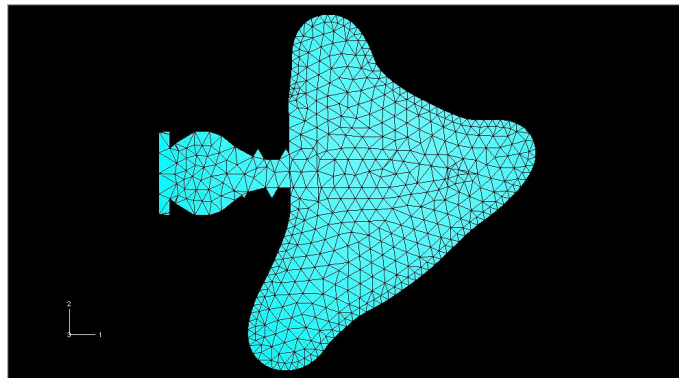
Figura 7 – Malha bi-dimensional de uma maxila atrófica e do MIO.
