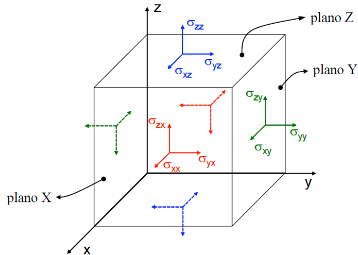
Figura 14 - Componentes de tensão atuando em um elemento cúbico infinitesimal
