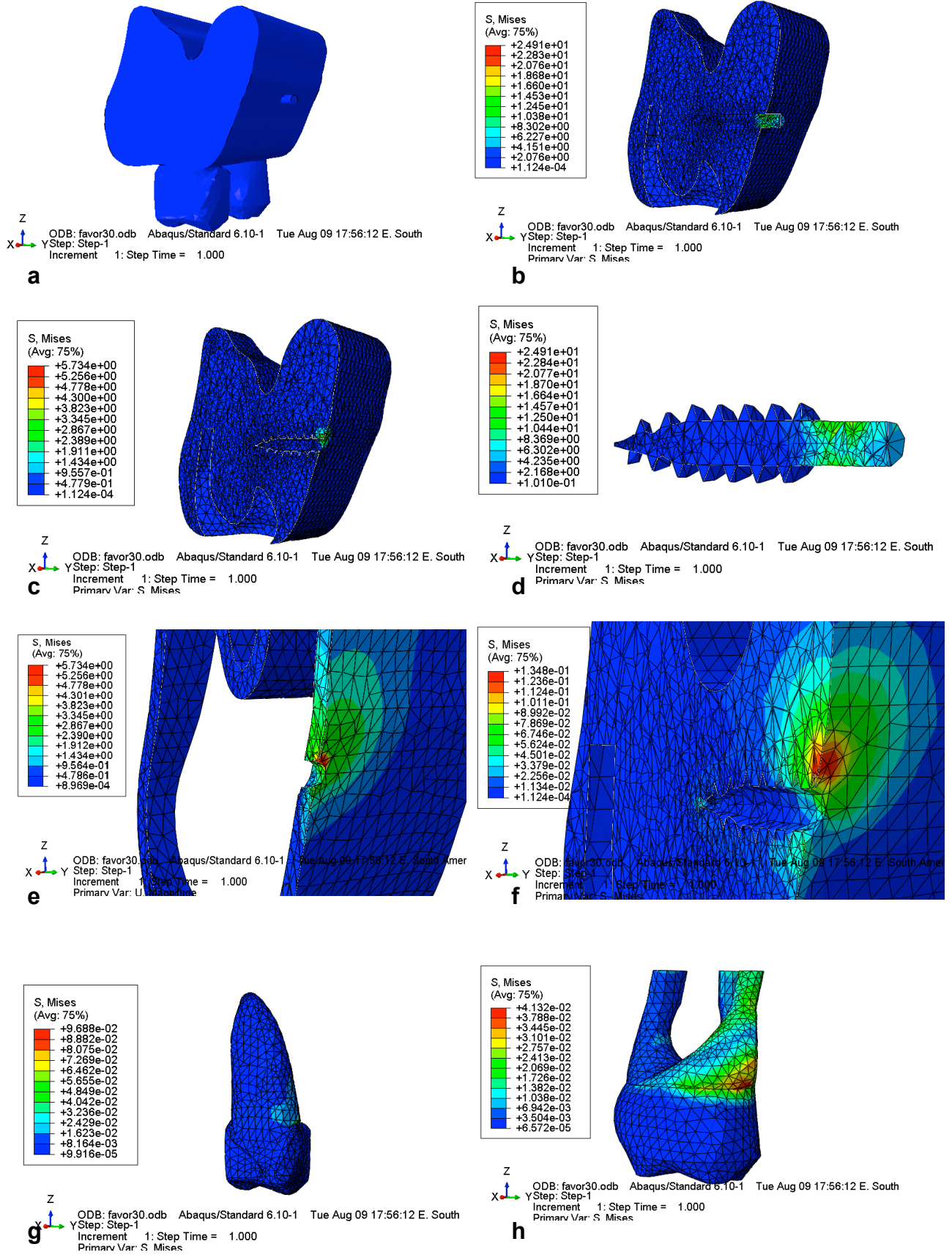
Figura 12 – Critério de von Mises para orientação de -30^\circ . Respectivamente: a) modelo completo; b) modelo completo seccionado; c) osso maxilar; d) MIO; e) osso cortical; f) osso medular; g) pré-molar; h) molar
